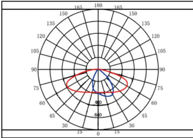
cd/klm — C0-C180, 151.8度 — C90-C270, 65.4度
